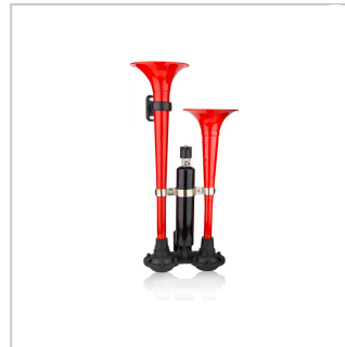
BÜYÜK İKİLİ HAVALI YANKILI KORNA (KIRMIZI)
